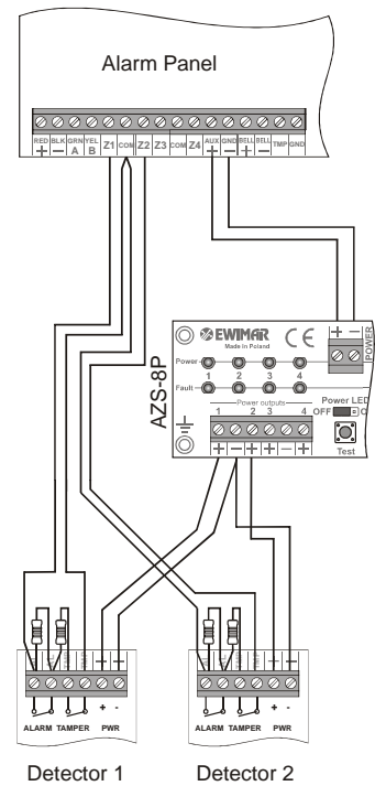
Separacja 8 linii zasilania czujek alarmowych
